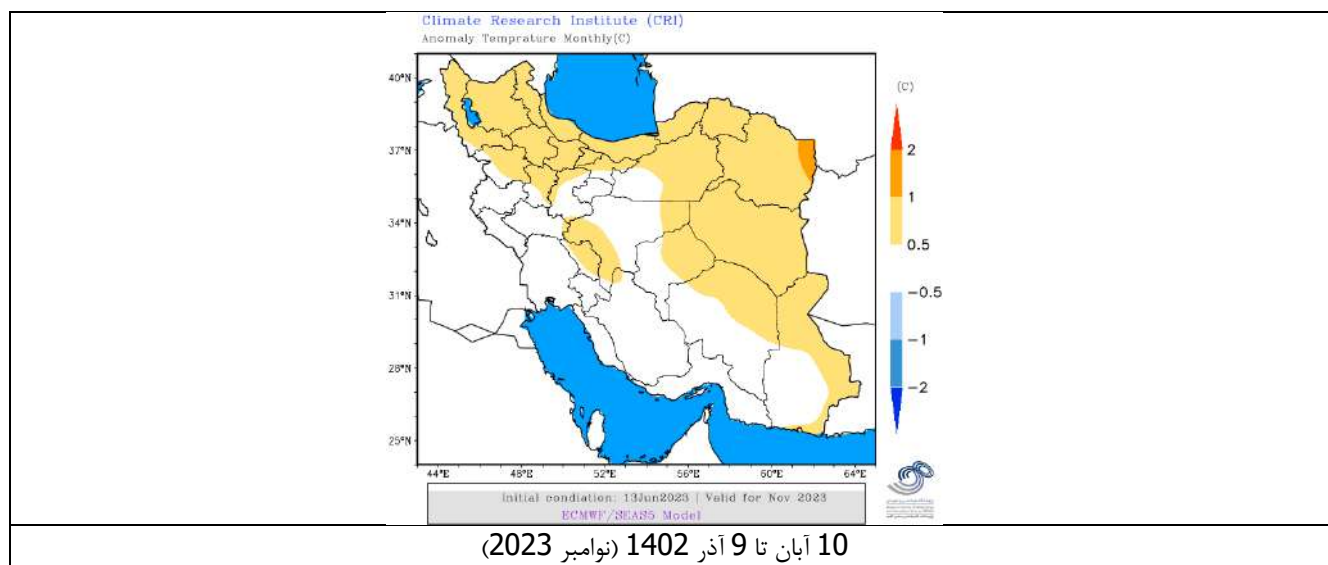
شکل : پیش‌بینی انحراف از نرمال دما از نیمه مرداد تا نیمه آذر 1402 (ژوئیه تا نوامبر 2023، از مدل ECMWF)
